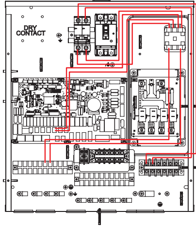
Met verwarmingsprintplaat
