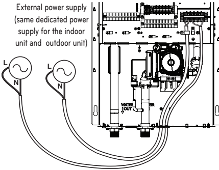
1Ø Elektrische kachel (Voor Hydrosplit)
