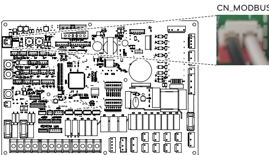
Indoorprintplaat
