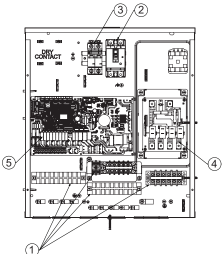
Met verwarmingsprintplaat
