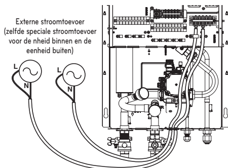
1Ø Elektrische verwarming (Voor R32)
