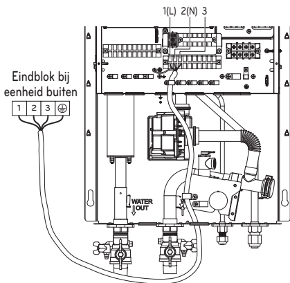
(Voor Hydrosplit)
