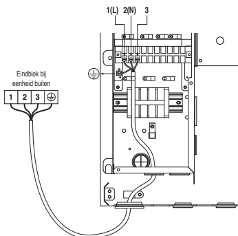
1Ø Elektrische verwarming
