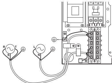
3Ø Elektrische verwarming
