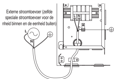
1Ø Elektrische verwarming
