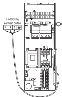
3Ø Elektrische verwarming
