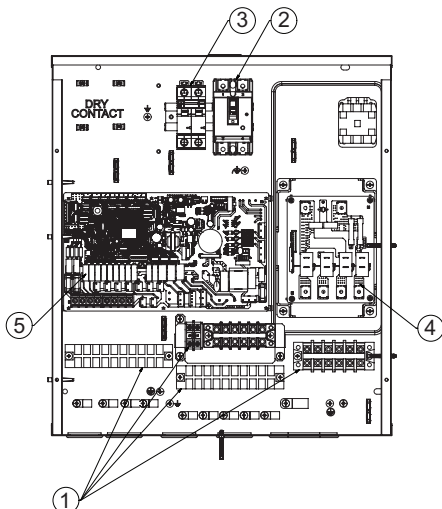
Met verwarmingsprintplaat (Datum : vanaf 1 okt. , 2019)
