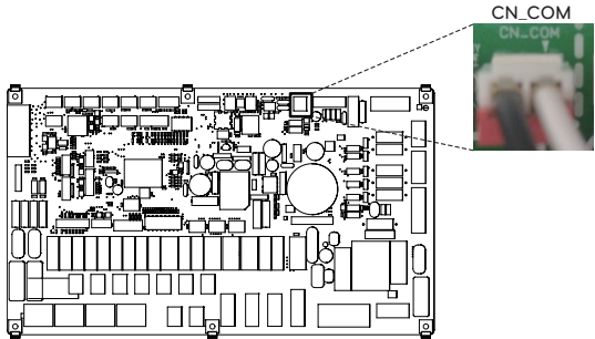
Indoorprintplaat
