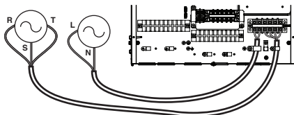
3Ø Elektrische kachel (Voor Hydrosplit)
