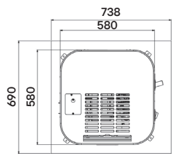
Bovenaanzicht
